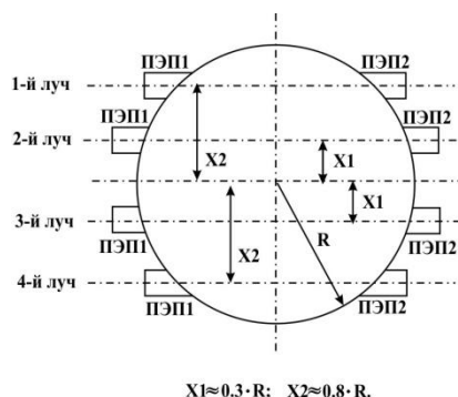
Рисунок 13 – Положение пар ПЭП для четырехлучевых расходомеров
