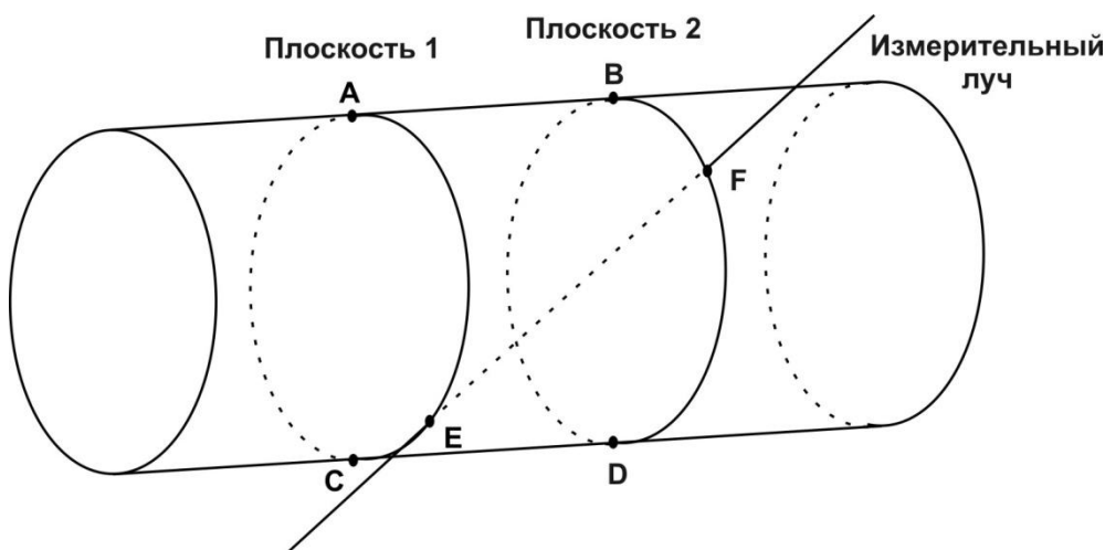
Рисунок 16 – Разметка заготовки УПР
