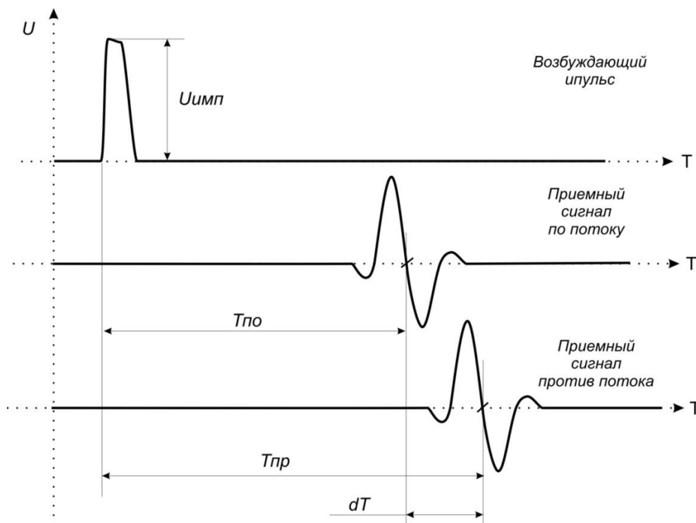
Рисунок 8 – Временные диаграммы ультразвуковых сигналов расходомера
